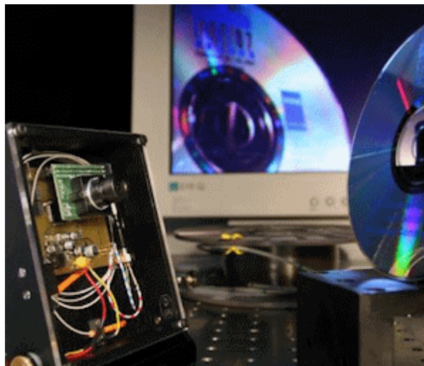
Die Kamera ist lediglich über ein Glasfaserkabel mit dem Rechner verbunden (Foto: kit.edu)
